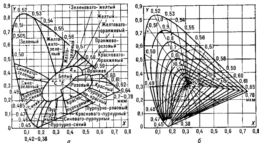
Рис. 6. Цветовой график системы XYZ: а — области цветностей в системе XYZ; б — линии постоянного цветового тона, чистоты цвета (сплошные) и насыщенности (пунктирные).
